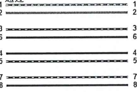
接线图 (T568B)
