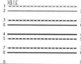
接线图 (T568B)
